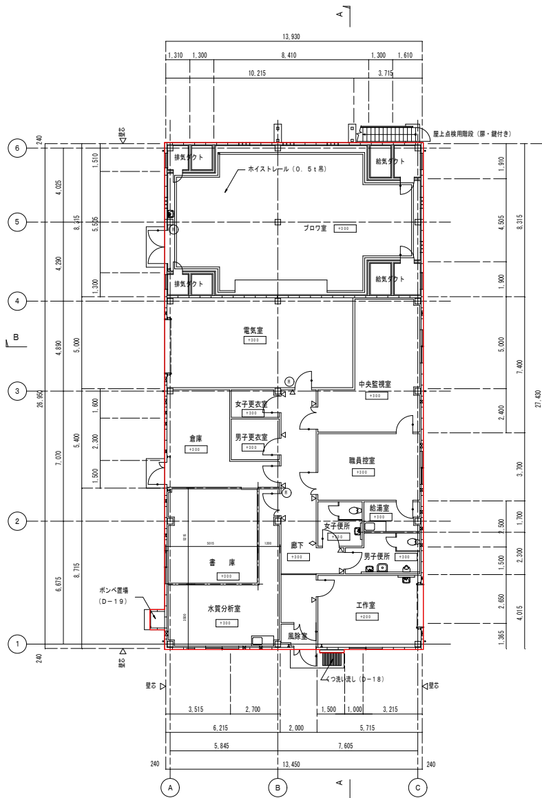
機械棟 平面図 1/100
