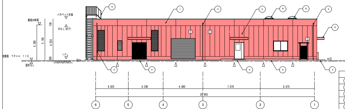
機械棟 西立面図 1/100
