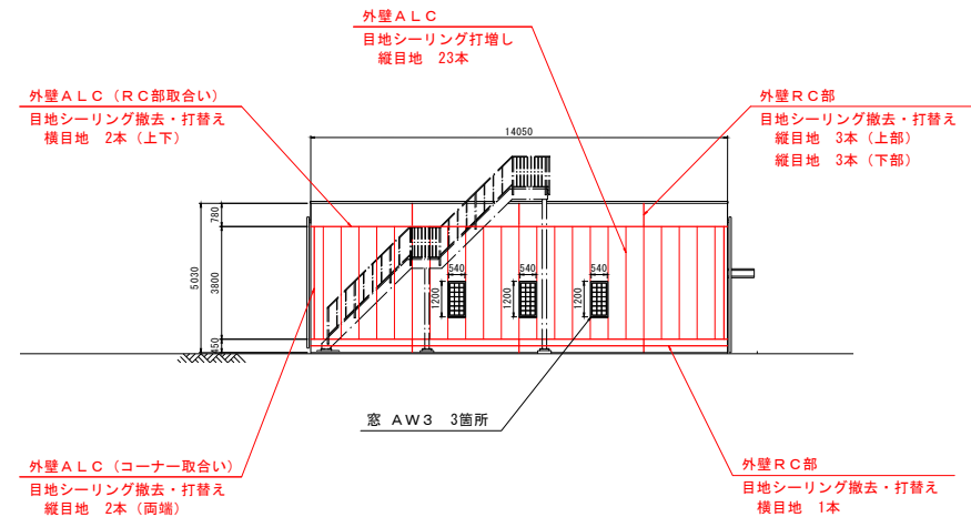
機械棟 北立面図 1/100
