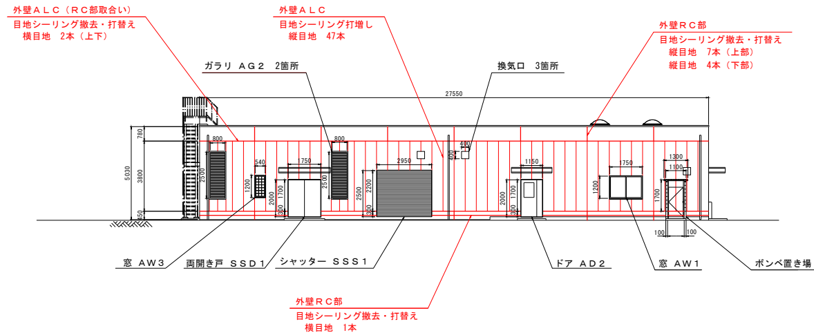
機械棟 西立面図 1/100
