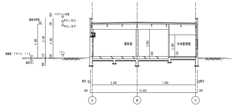
機械棟 B-B断面図 1/100
