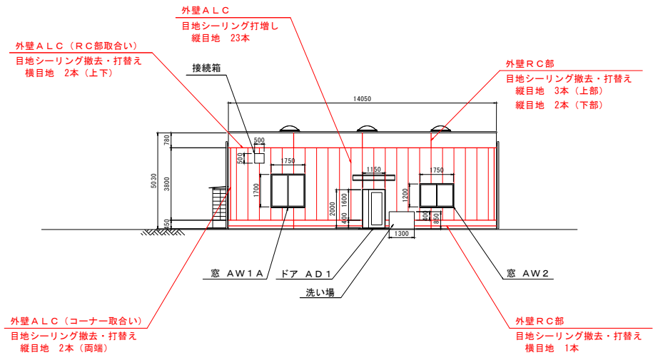
機械棟 南立面図 1/100
