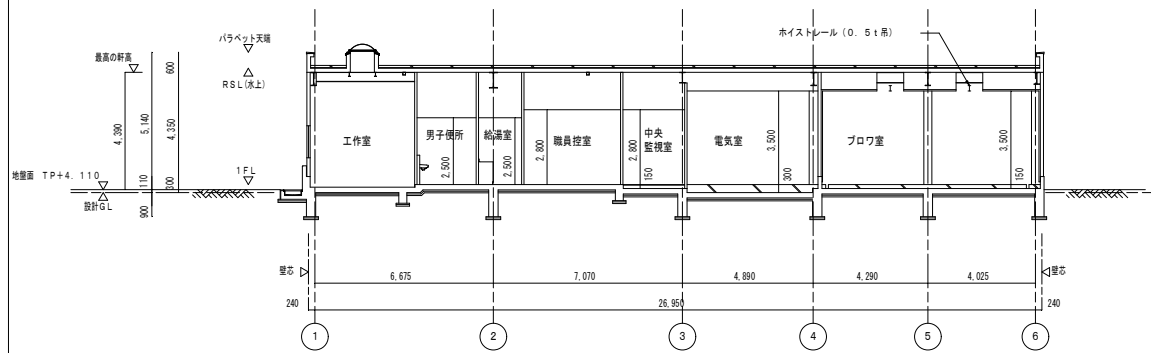
機械棟 A-A断面図 1/100
