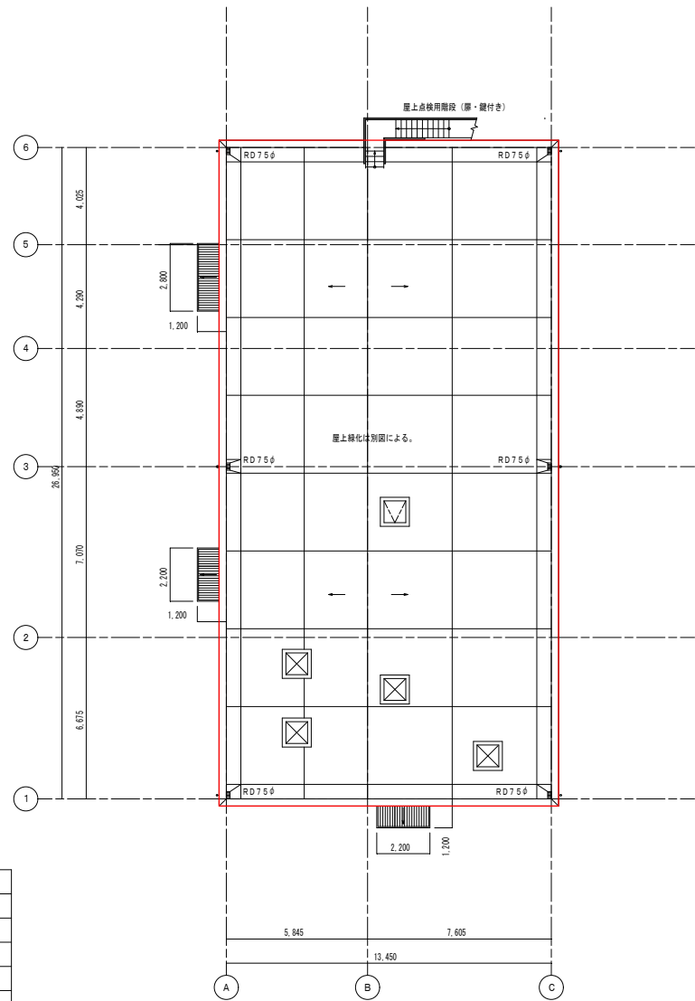
機械棟 屋根伏図 1/100
