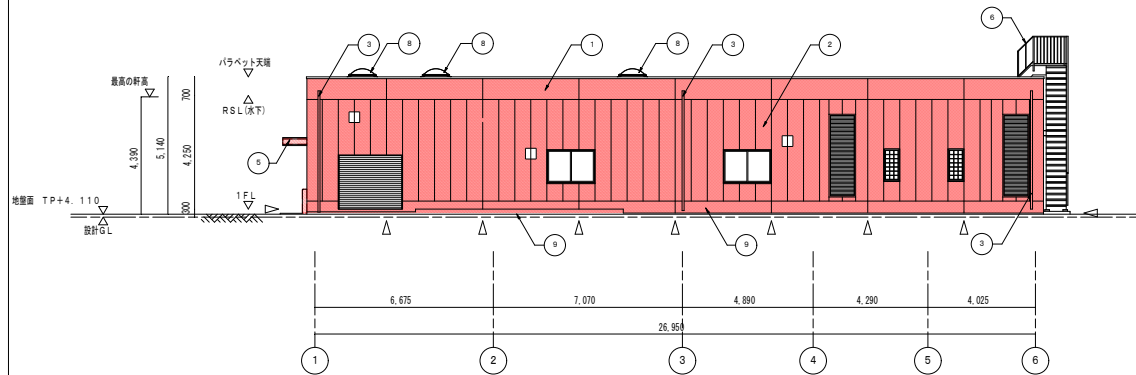
機械棟 東立面図 1/100
