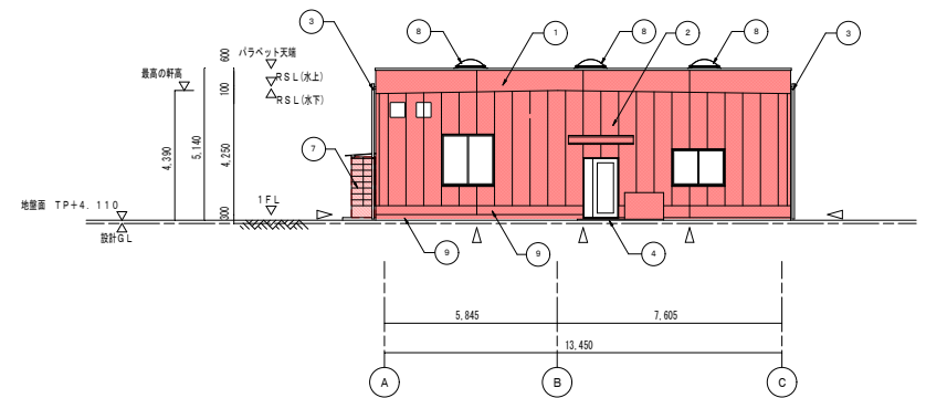
機械棟 南立面図 1/100
