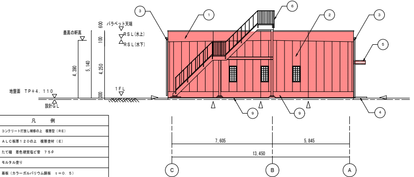
機械棟 北立面図 1/100
