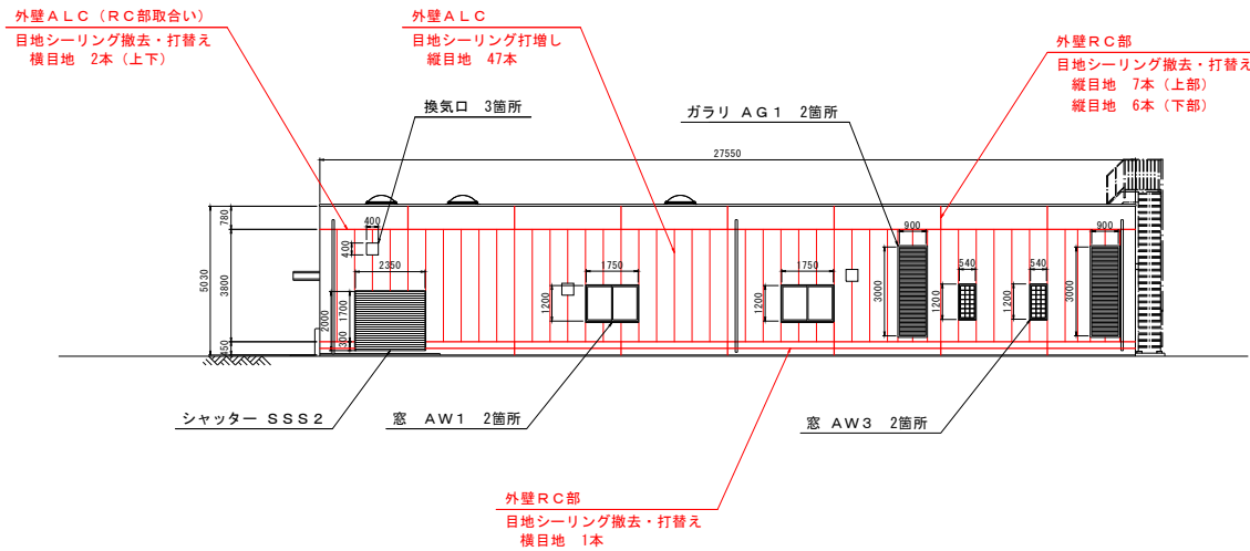
機械棟 東立面図 1/100
